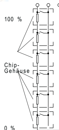
Внутренняя схема датчика уровня
