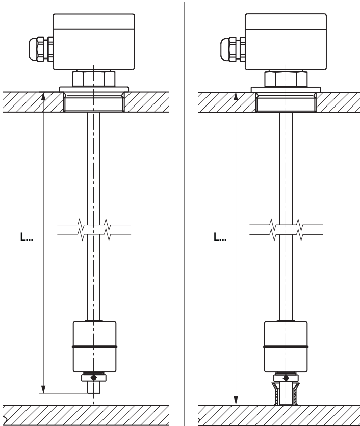
Вариант А Крепление прибора на крыше бака
